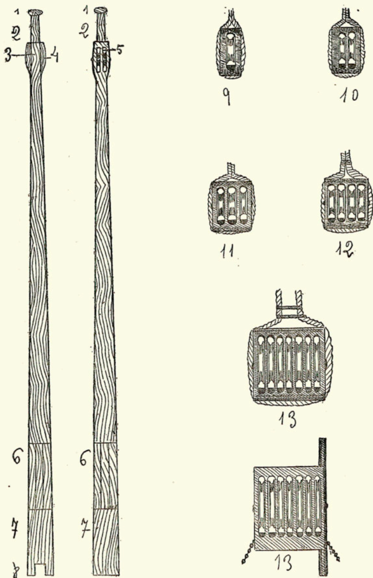
1. Galeta. — 2. Espigó. — 3. Calcés. — 4. Vas. — 5. Granera. — 6. Afogament. — 7. Culata. — 8. Metxa. — 9. Bussell. — 10. Bussell doble. — 11. Ternal. — 12. Quadernal. — 13. Guindares.
