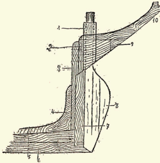
1. Tremuja del timó. — 2. Dragant vertical. — 3. Contraroda. — 4. Corba coral. — 5. Sobrequilla. — 6. Quilla. — 7. Codast. — 8. Timó. — 9. Dragant horizontal. — 10. Gambota.
