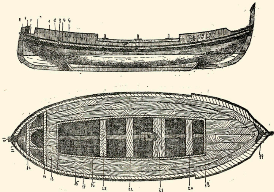
BARCA DE PALANGRA
